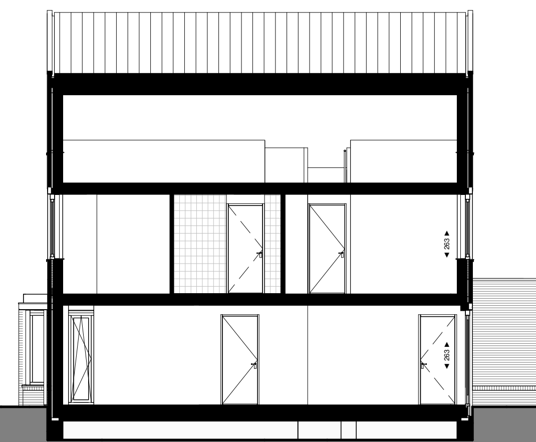
Doorsnede B
