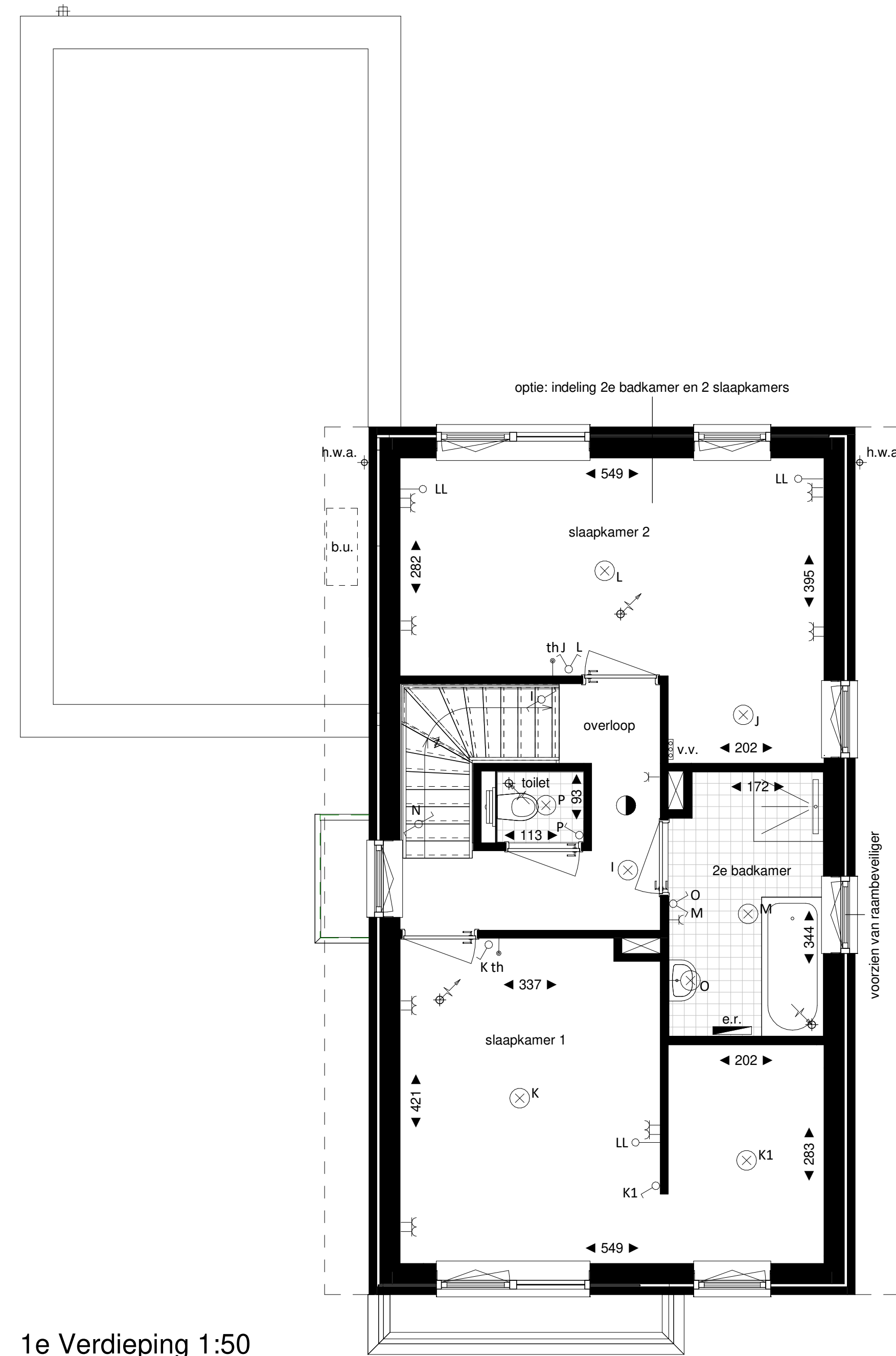
1e Verdieping 1:50
