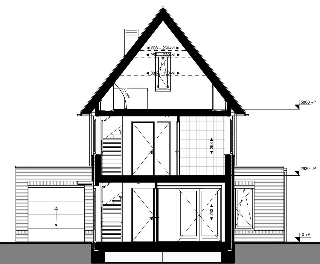
Doorsnede A
