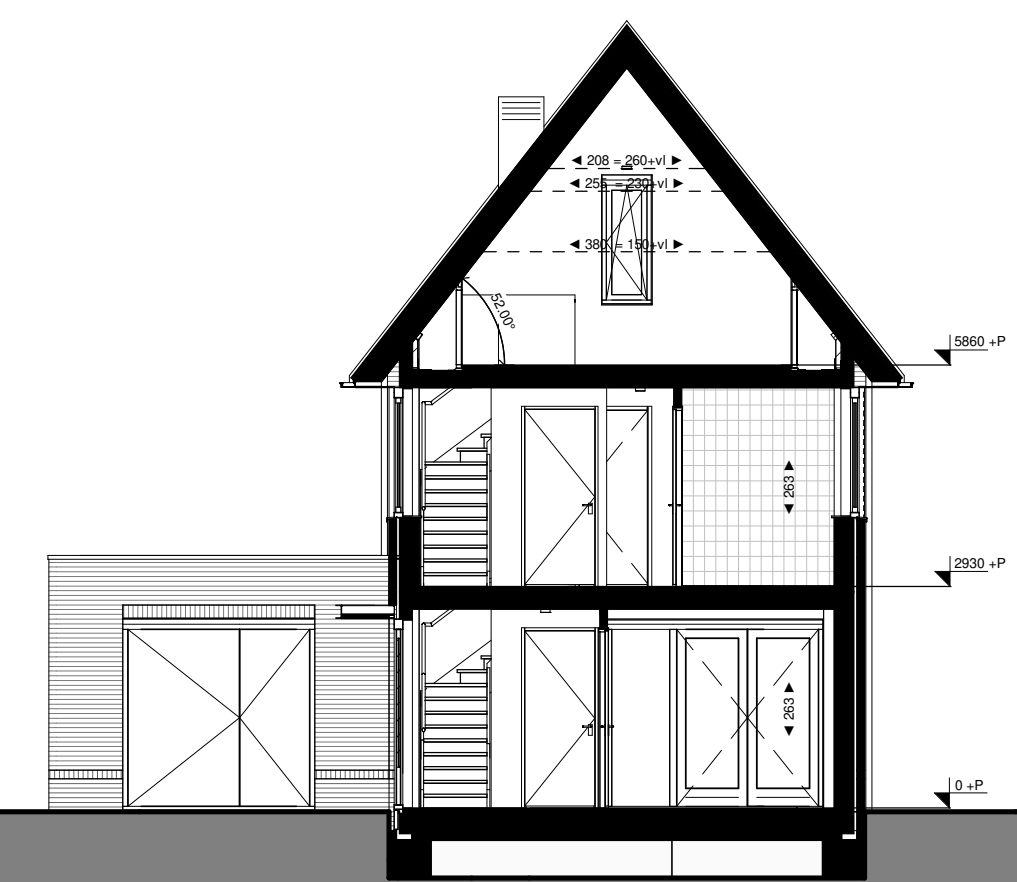
Doorsnede A
