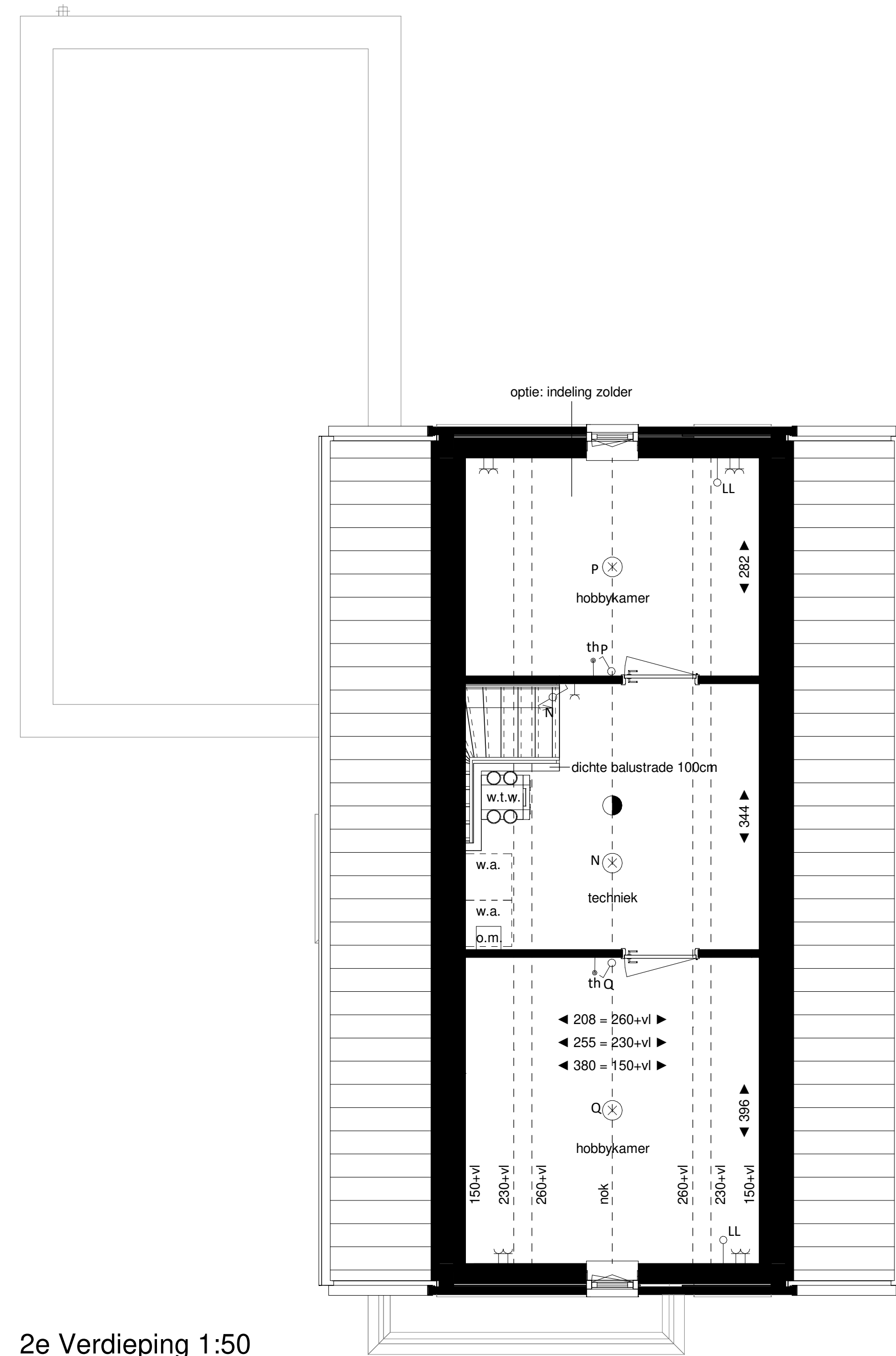
2e Verdieping 1:50
