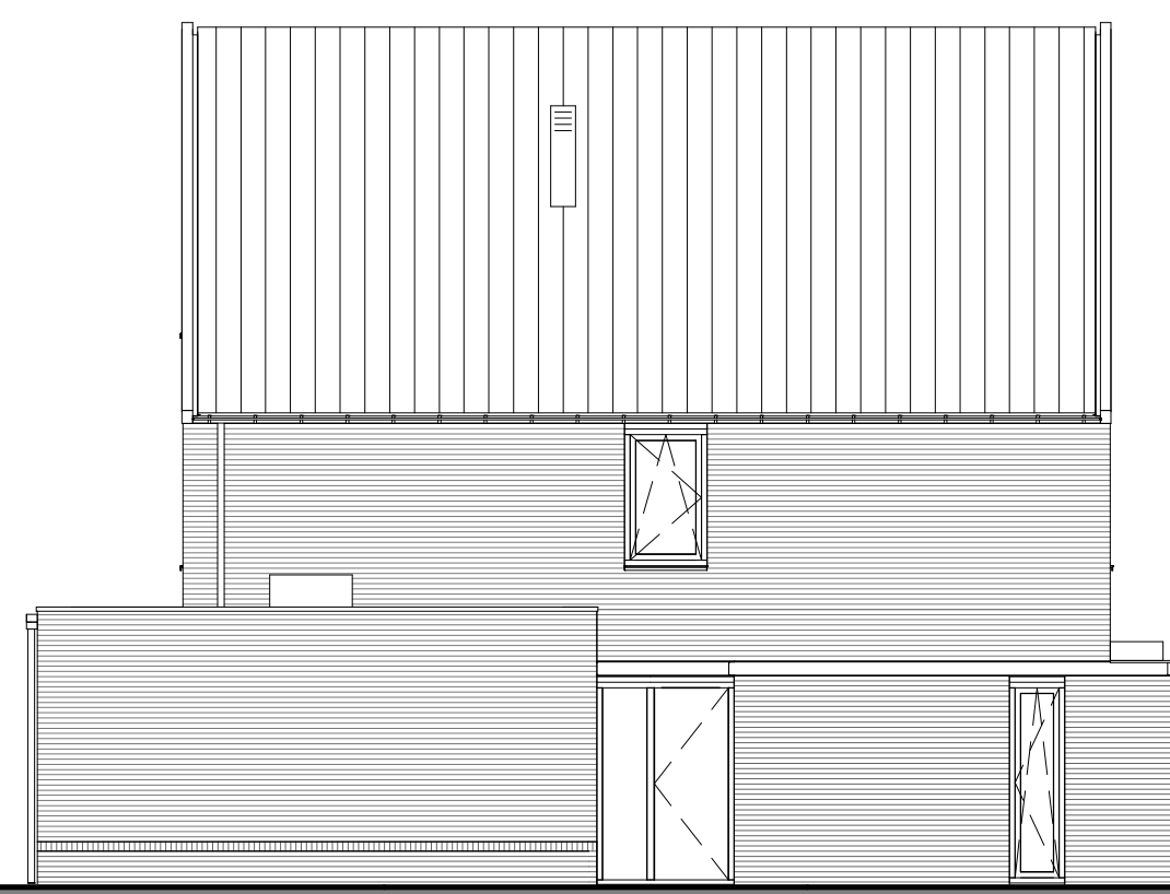
Linker zijgevel
