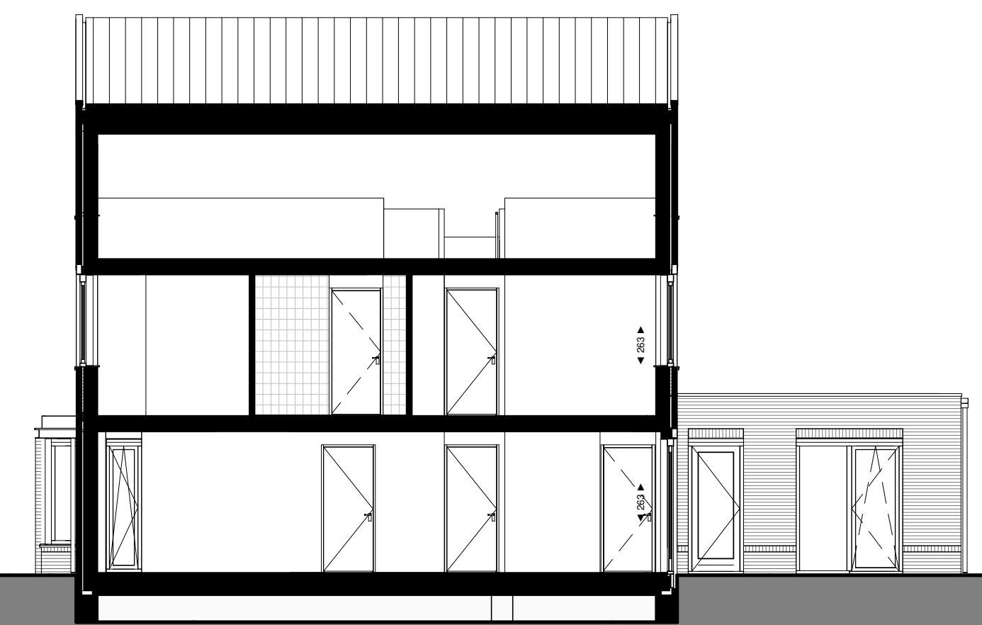
Doorsnede B
